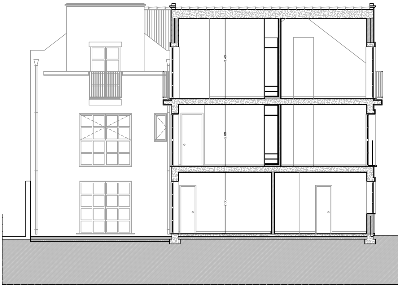
CORTE AB
